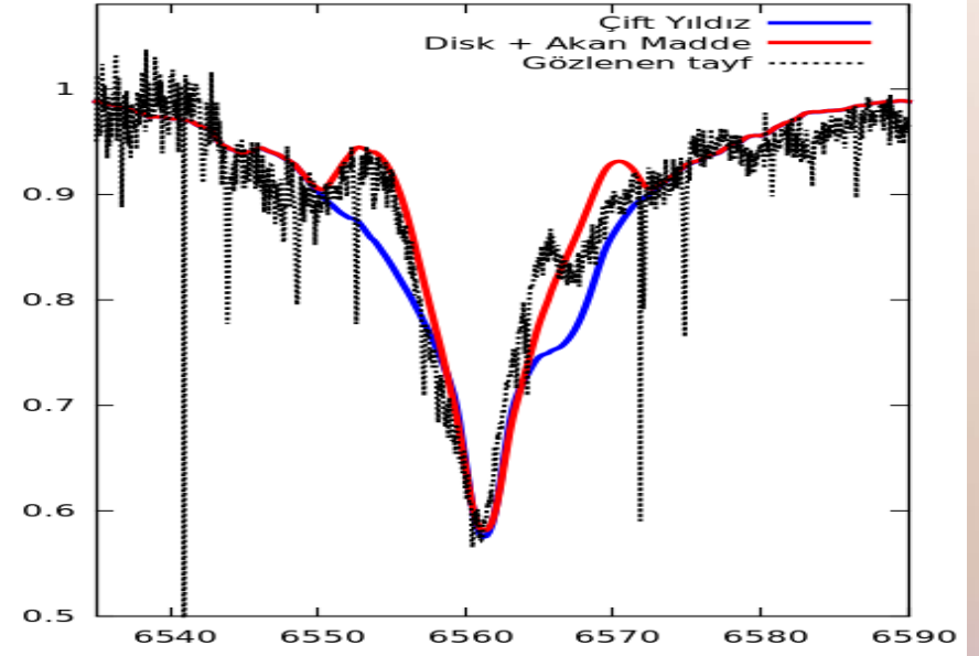
U Sge, evre=0.25
