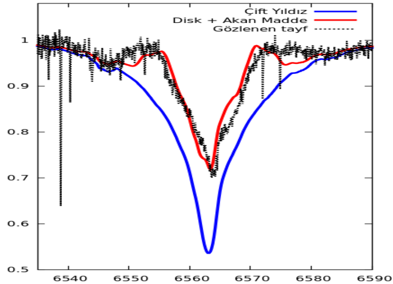
U Sge, evre=0.54
