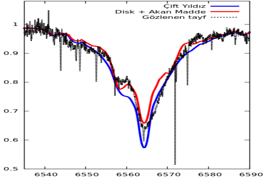
U Sge, evre=0.75
